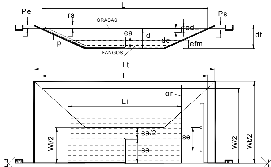
PLANTA LAGUNA ANAEROBIA
