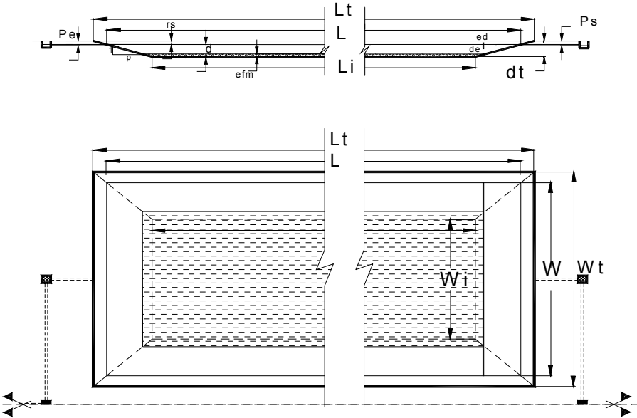
LAGUNA AIREADA DE MEZCLA TOTAL
