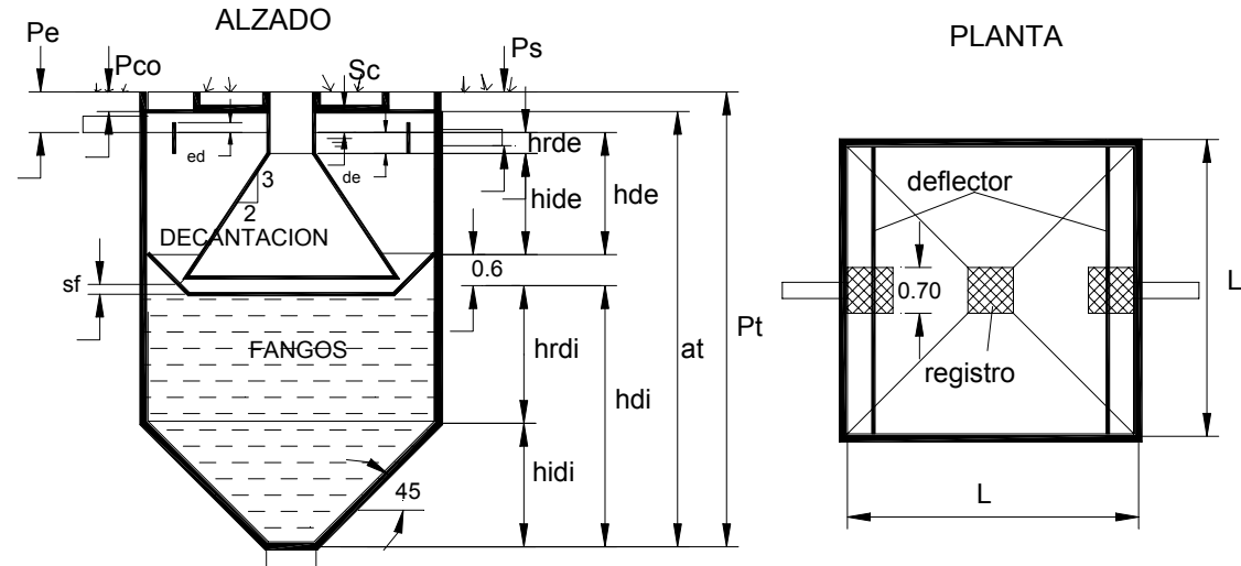
TANQUE IMHOFF CUADRADO
