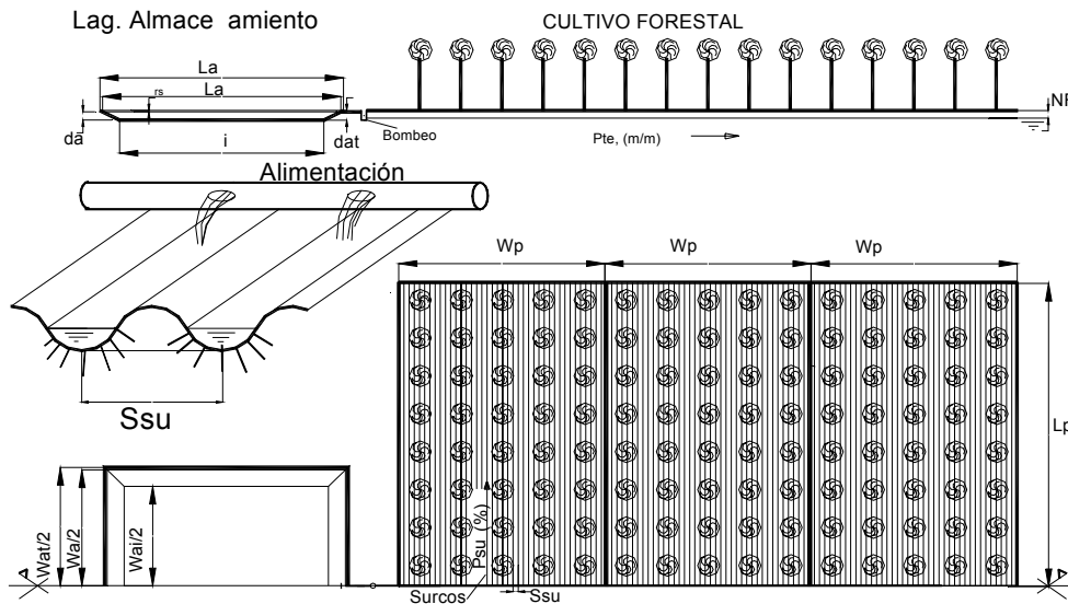
RIEGO FORESTAL SUPERFICIAL
