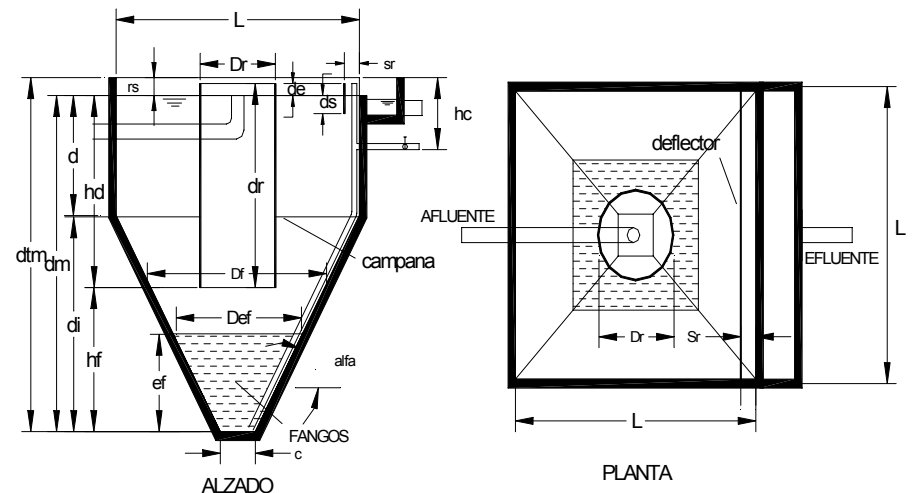
DECANTADOR ESTATICO CUADRADO
