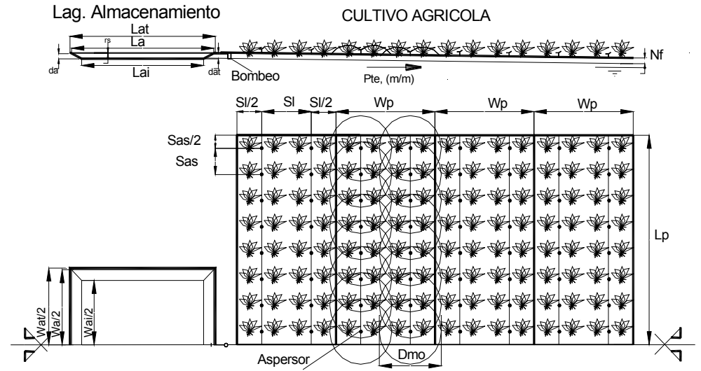
RIEGO AGRICOLA POR ASPERSION
