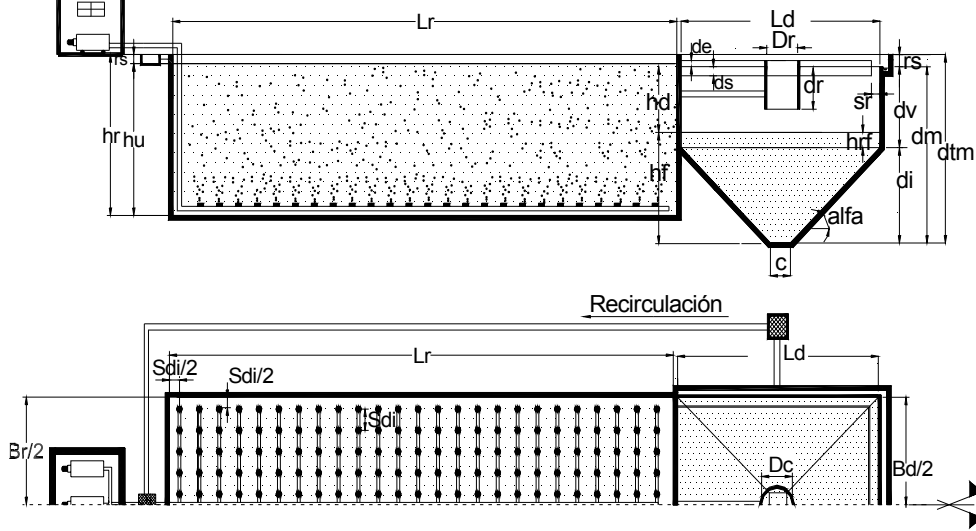
Soplante REACTOR CON DIFUSORES DISCO DECANTADOR ESTATICO RECTANGULAR
