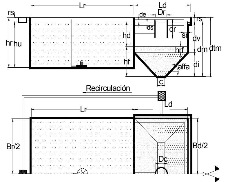
REACTOR AIREADORES SUMERGIDOS DECANTADOR ESTATICO RECTANGULAR
