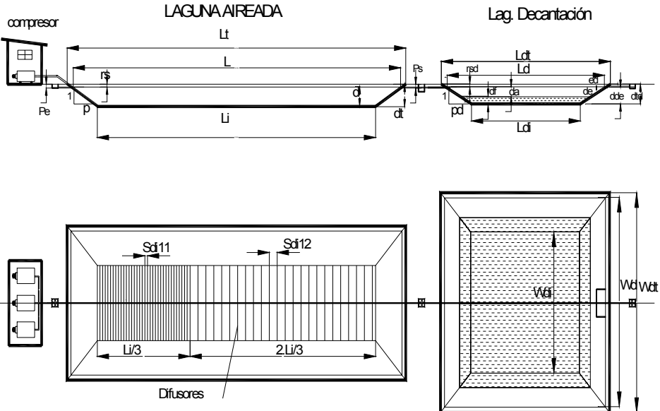
LAGUNA AIREADA MEZCLA TOTAL
