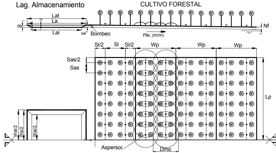
RIEGO FORESTAL POR ASPERSION
