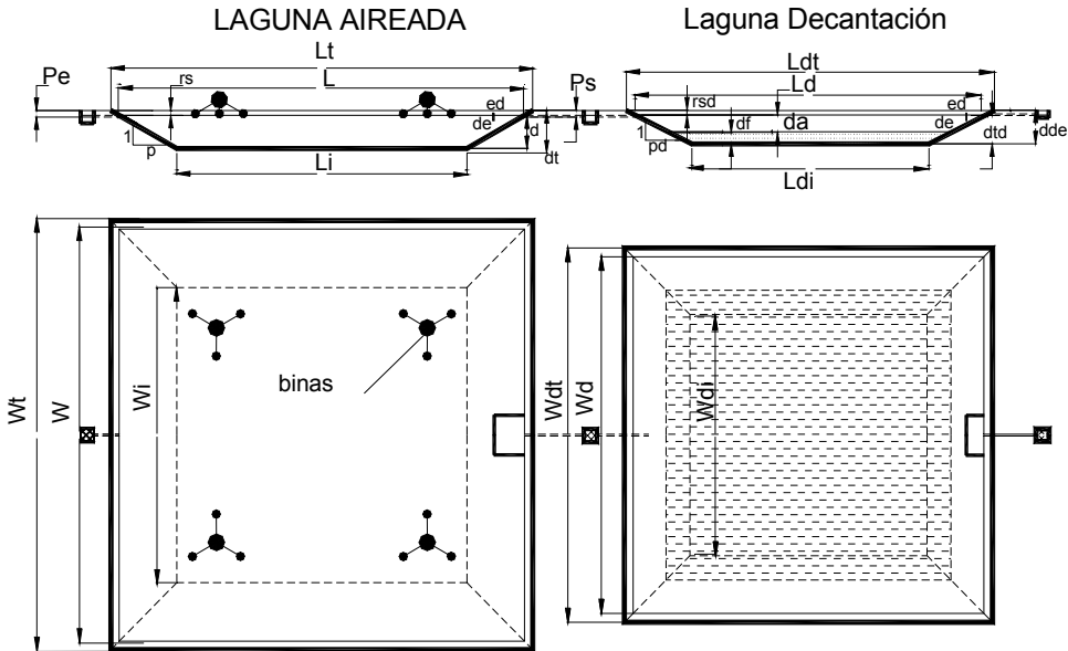
LAGUNA AIREADA DE MEZCLA TOTAL
