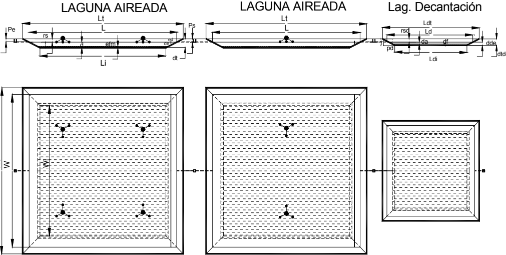
LAGUNA AIREADA MEZCLA TOTAL
